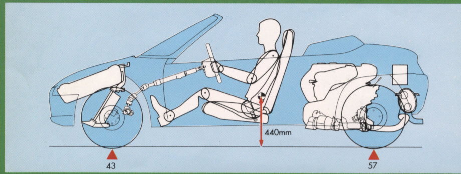
理想の前後重量配分と低重心を実現
