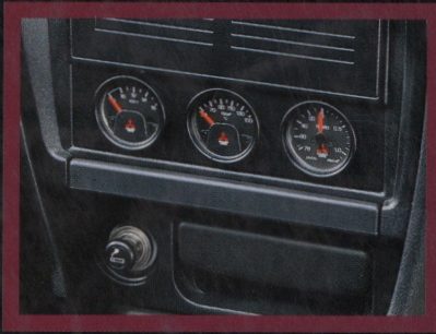
⑬ スポーツメーターキット 油温計/電圧計/ターボ計の3連メーター。 MZ605828 ¥57,500(参考取付工賃¥12,500含む) *ターボ計はバキュームメーターを組み込んだ連成タイプ。ターボ・オフ時は、マニホールド負圧を示します。
