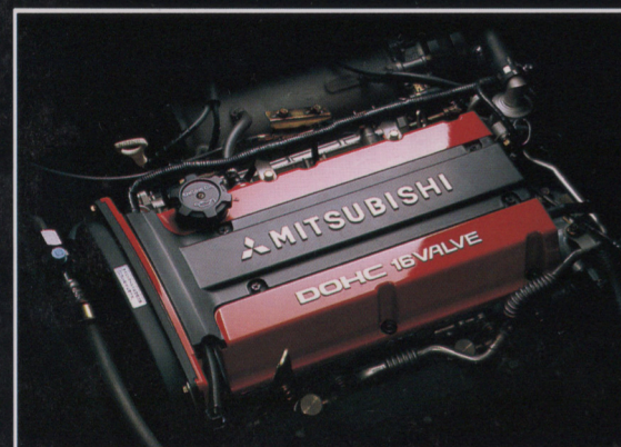
2000DOHC 16V I/C T/C エンジン
