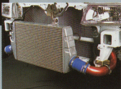
写真は装着イメージです。(ストラットタワーバーはオプション)
