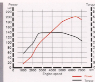
GT-A性能曲線図
