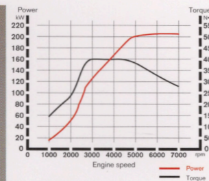
GSR性能曲線図
