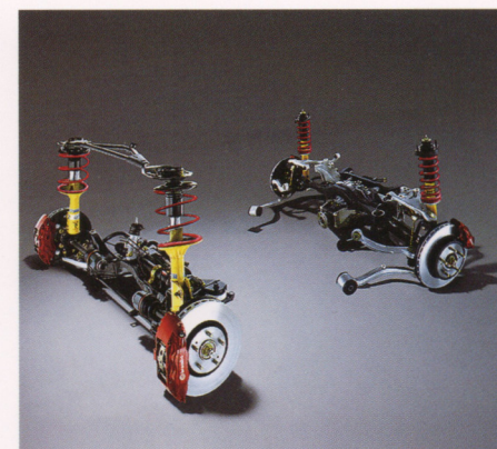
サスペンション(フロント: マクファーソンストラット式、リヤ: マルチリンク式)
