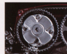
MIVEC [連続可変バルブタイミング] システム
