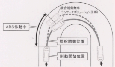
ACD+スーパーAYC+スポーツABS統合制御
