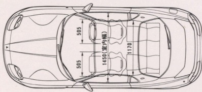
'94-'95日本カー・オブ・ザ・イヤー受賞記念限定車 外観図(単位=mm)
