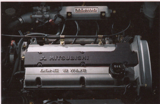
MAX. POWER (最高出力・ネット) 205PS/6000rpm MAX. TORQUE (最大トルク) 28.0kg-m/3000rpm
