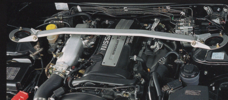
■SR20DETチューンドエンジン+専用フロントストラットタワーバー
