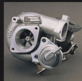
■専用ターボチャージャー (IHI製)
