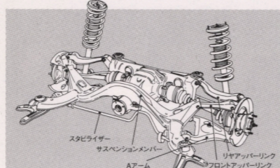
リヤマルチリンクサスペンション
