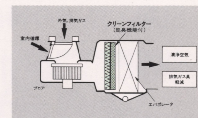
クリーンフィルター(脱臭機能付)
