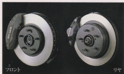
4輪アルミキャリパー対向ピストンブレーキ
